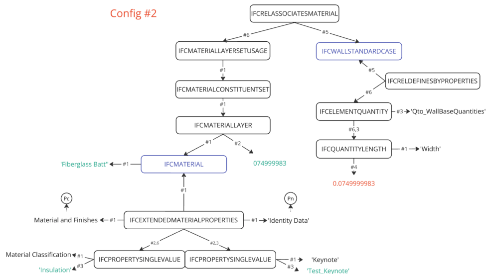
Figure 3. Schéma illustratif de l'association entre les différents niveaux IFC2×3-Revit
